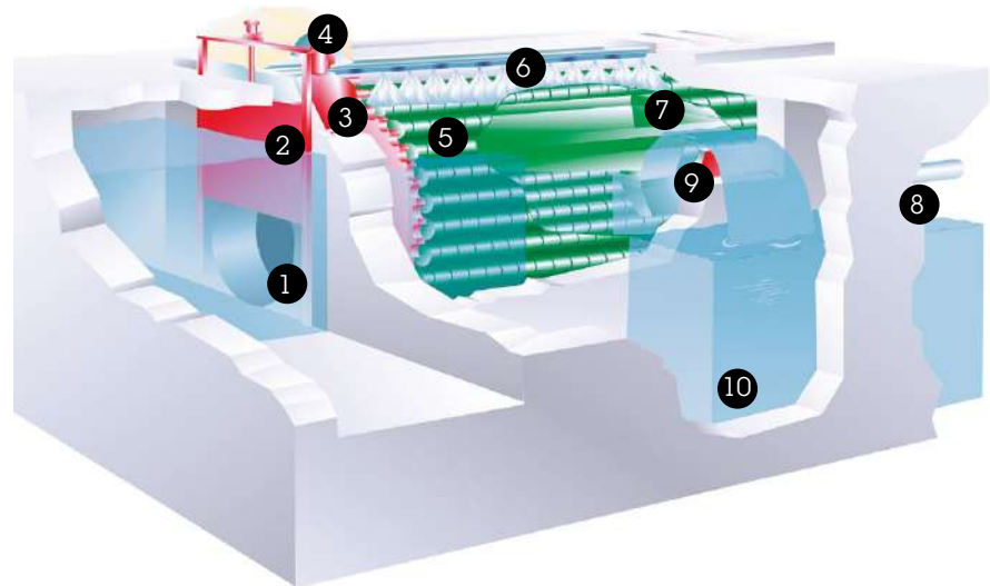
Funktionsablauf Trommelsieb RSH-M
